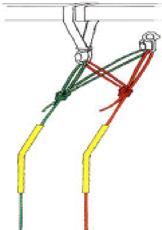
Figura 32. Ancoragens independentes.
